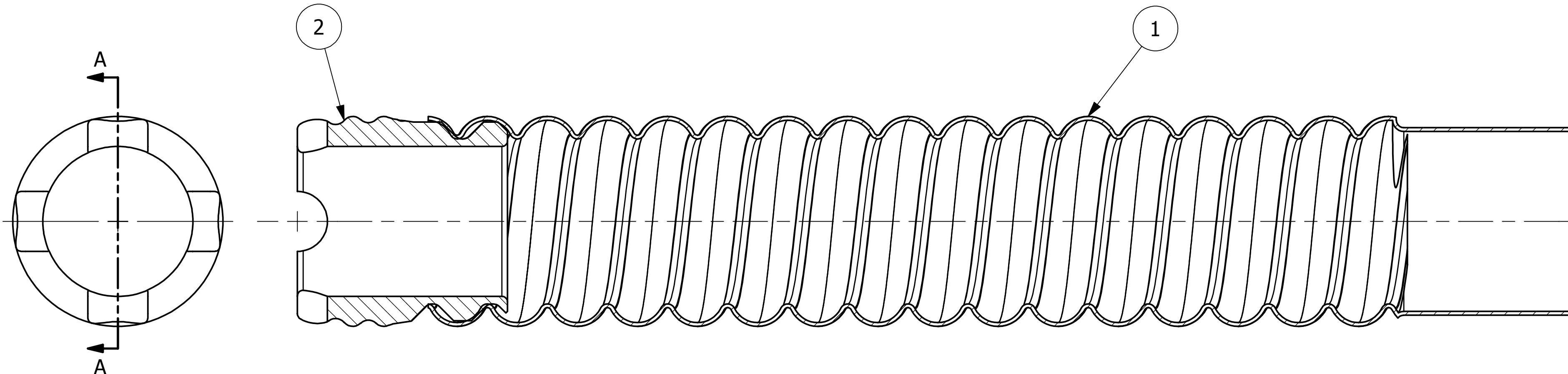
SECTION A-A
