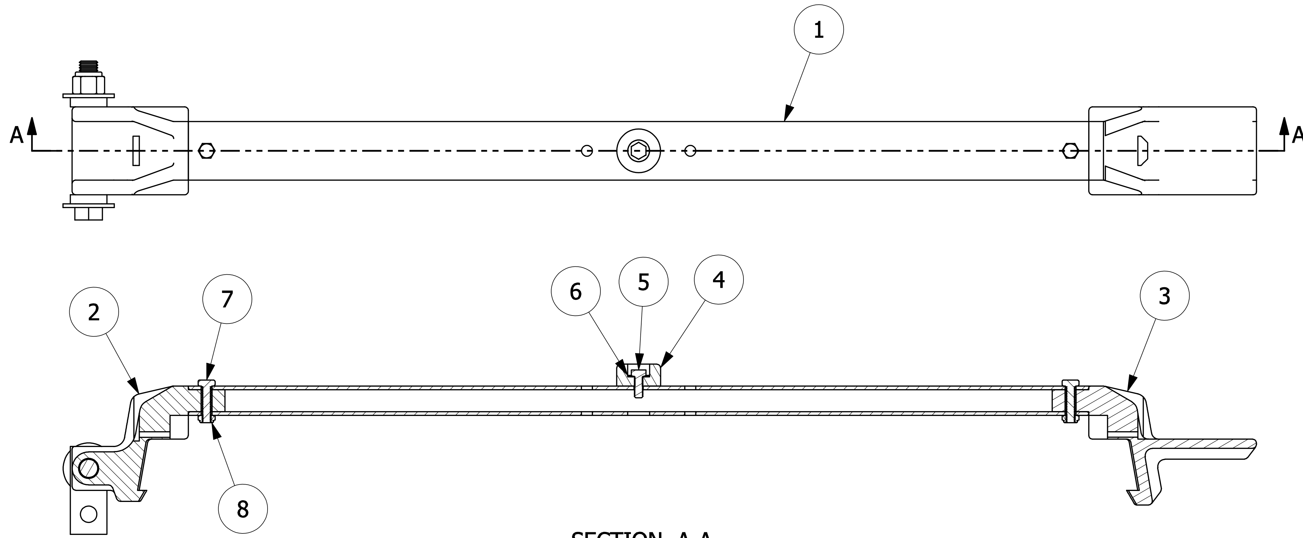
SECTION A-A
